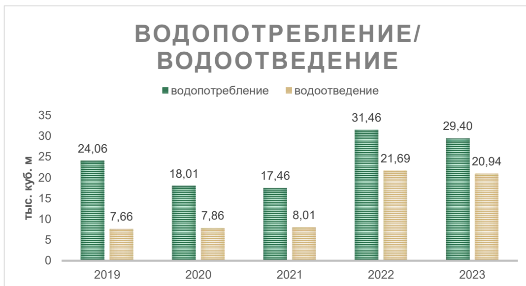
Рисунок 3. Водопотребление и водоотведение за период 2019-2023гг.
