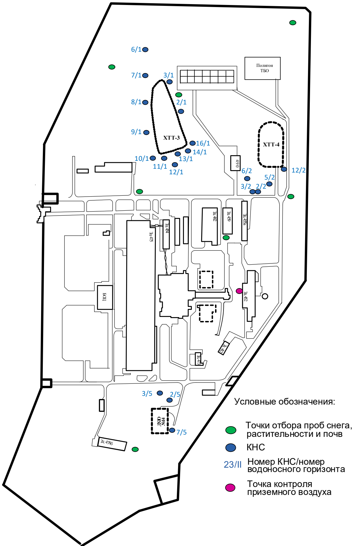
Рисунок 2. Площадка 11. Точки отбора проб
