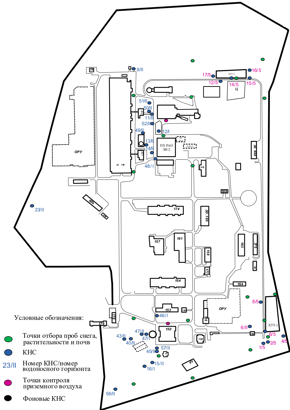
Рисунок 1. Площадка 2. Точки отбора проб
